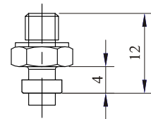
EN-PB-13~15-M5
