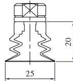
SBME-25-1/8W
