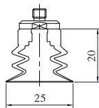
SBME-25-M5
