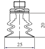
SBME-25-1/8M
