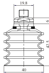
SBLE-40-1/8M
