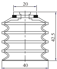
SBLE-40
