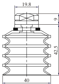
SBLE-40-1/8W
