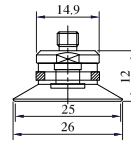
SFE-25-M5
