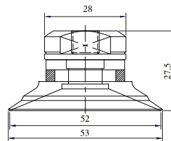
SFE-50-1/8W SFE-50-1/4W
