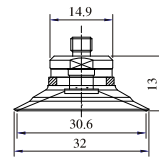
SFE-30-M5
