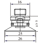
SFE-25-1/8M
