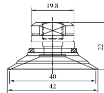
SFE-40-1/8W
