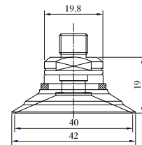
SFE-40-1/8M
