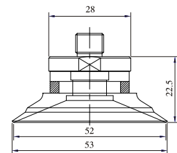
SFE-50-1/8M SFE-50-1/4M
