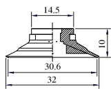
SFE-30
