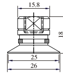
SFE-25-1/8W
