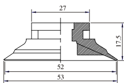
SFE-50
