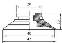
SFE-40
