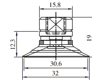
SFE-30-1/8W
